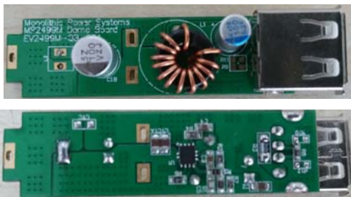
(L x W x H) 5.5cm x 1.4cm x 1.1cm (Two layer PCB)
