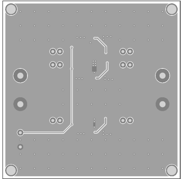
Figure 2—Bottom Layer
