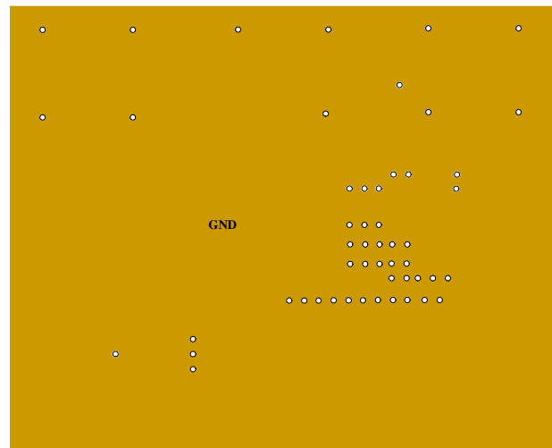
Inner1 Layer
