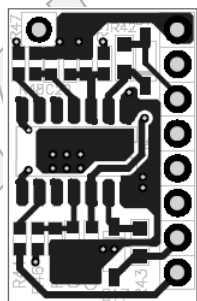
Figure 1—Top Layer
