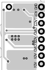
Figure 2—Bottom Layer
