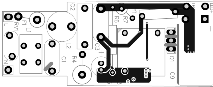
Figure 2—Top Layer
